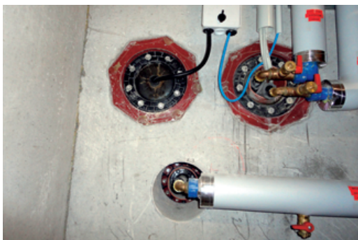
RDS-Rohrdurchführungssysteme
